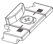
A-01090-00-0-1 Alu-System Adjustable Locking Plate
